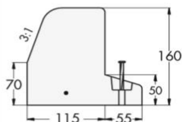
Snitt tegning Kantstein D
